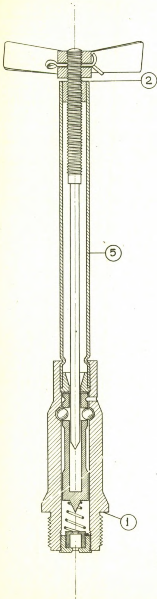
FUZE N. 1.
