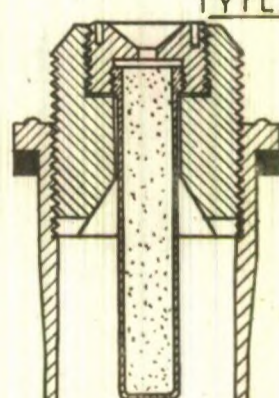
TYPE F.
