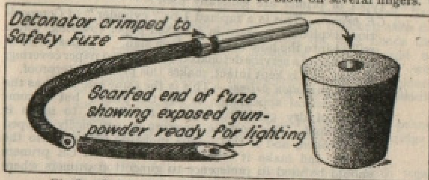
Fig 2. Safety fuze, No. 27 detonator and 1 oz. primer
