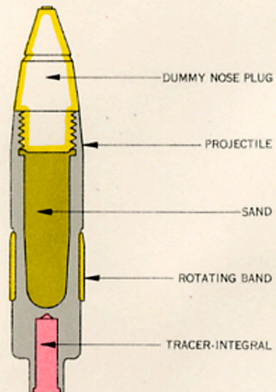
FIG. 3.—TARGET
