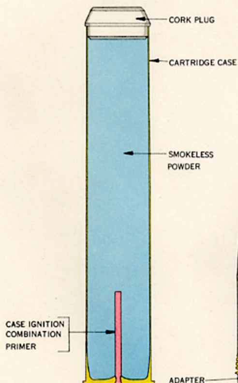
FIG. 1.—CARTRIDGE
