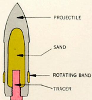
FIG. 2.—TARGET
