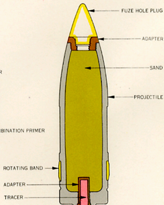
FIG. 3.—TARGET
